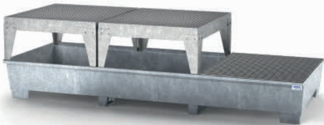
Typ 3 verzinkt mit Gitterrost und zwei Abfüllböcken
